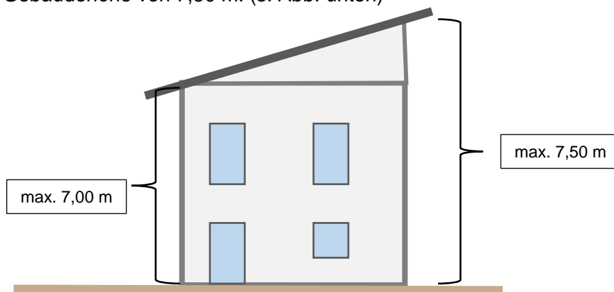
Abbildung: Gebäudehöhenregelung einhüftiges Pultdach ohne Staffelgeschoss | BBP
